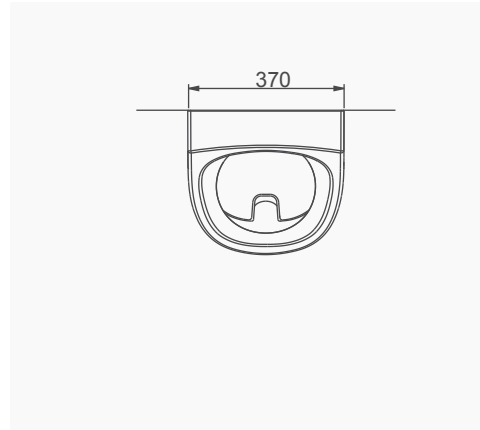
A052 NATURA ARKADAN ÇIKIŞLI KLOZET / NATURA P-TRAP CLOSE-COUPLED WC A051002 KLOZET / WC PAN A052001 REZERVUAR (İç Takımsız) / CISTERN (Without Flush Mechanism) A055001 NATURA KLOZET KAPAĞI / NATURA STANDART WC SEAT & COVER
