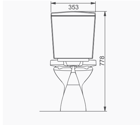
A051 NATURA ALT TAN ÇIKIŞLI KLOZET / NATURA S-TRAP CLOSE-COUPLED WC A051001 KLOZET / WC PAN A052001 REZERVUAR (İç Takımsız) / CISTERN (Without Flush Mechanism) A055001 NATURA KLOZET KAPAĞI / NATURA STANDART WC SEAT & COVER
